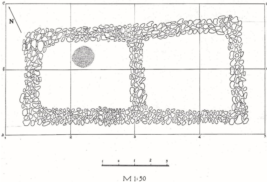
Фиг. 6. План на гробница 2/III (Торбов, Н. Могиланската могила във Враца, Враца, 2005, с.19,обр.2)
